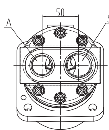
насос правый
