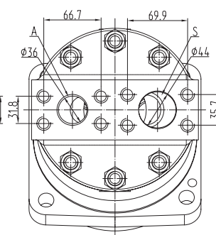
насос правый
