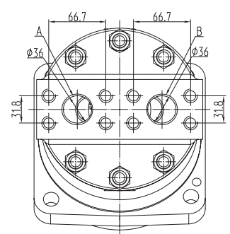
гидромотор
