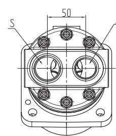
насос левый
