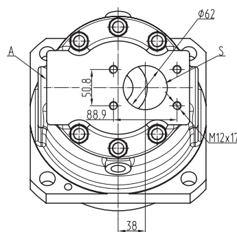
насос правый
