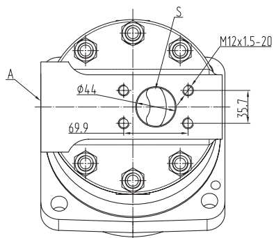
насос правый
