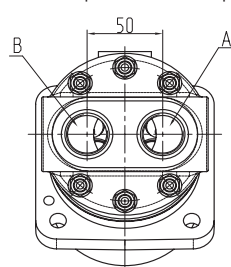
гидромотор
